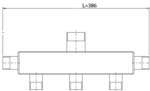
Rett manifold - målskisse
