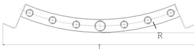
Buett manifold - målskisse
