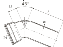
S-9674 Muffespiss bend 45°
