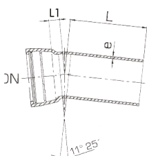
S-9674 Muffespiss bend 11 1/4°
