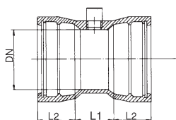
S-9171 Dobbeltmuffe m gjengeavstikker 2 "
