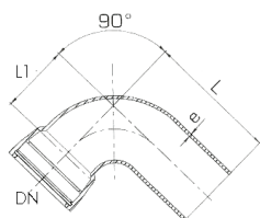
S-9674 Muffespiss bend 90°
