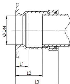
S-9170-5 Flensemuffe kort
