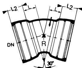
S-9175 Tyton bend 30° Med to muffer
