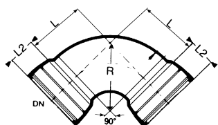
S-9175 Tyton bend 90° Med to muffer
