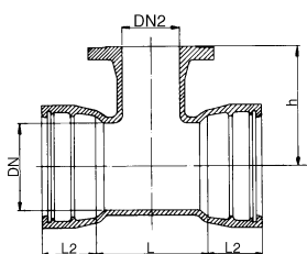
S-9178 Dobbelmuffe Med flenseavstikker
