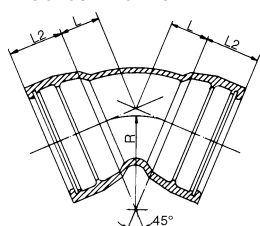
S-9175 Tyton bend 45° Med to muffer
