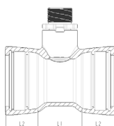
S-9121 Dobbeltmuffe m/Esco Lock* Bajonettkobling i avsinkningsfri messing Med 2 " utv og 1 ½ innvendige rørgjenger
