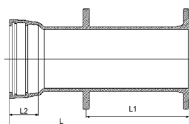
S-9173-14 Veggjennomgang Med flensekrage
