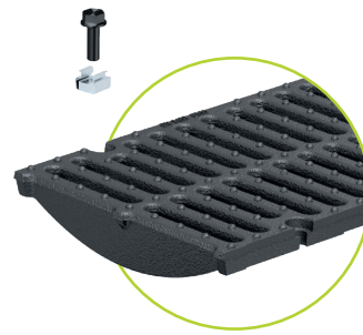
6 SPALTERIST I STØPEJERN spaltebredde 14/95, klasse F
