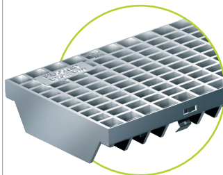
2 GITTERIST MW 25/10 klasse D Galvanisert stål.
