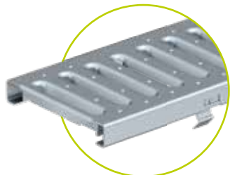
1 SPALTERIST SW 8/80 klasse A 15 – C 250 Galvanisert stål.
