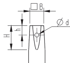
Dimensjoner spindeltopp:
