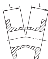
S-9668 Flensebend 30°
