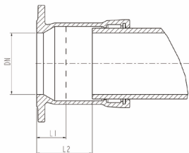
S-9170-5 Flensemuffe kort
